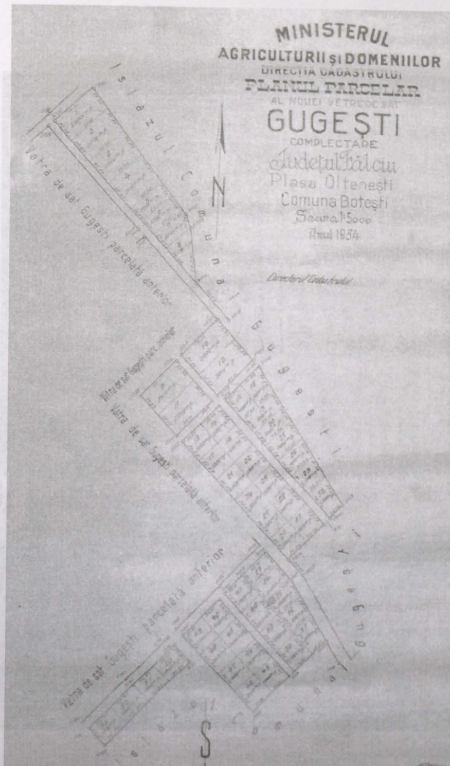
Planșa nr. 2 – Planul parcelar al noii vetre de sat Gugești. Complectare – 1934
